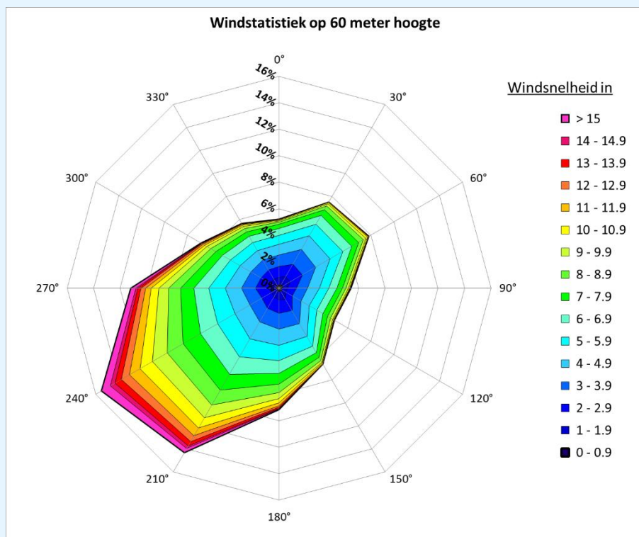
figuur 5: windstatistiek plangebied
