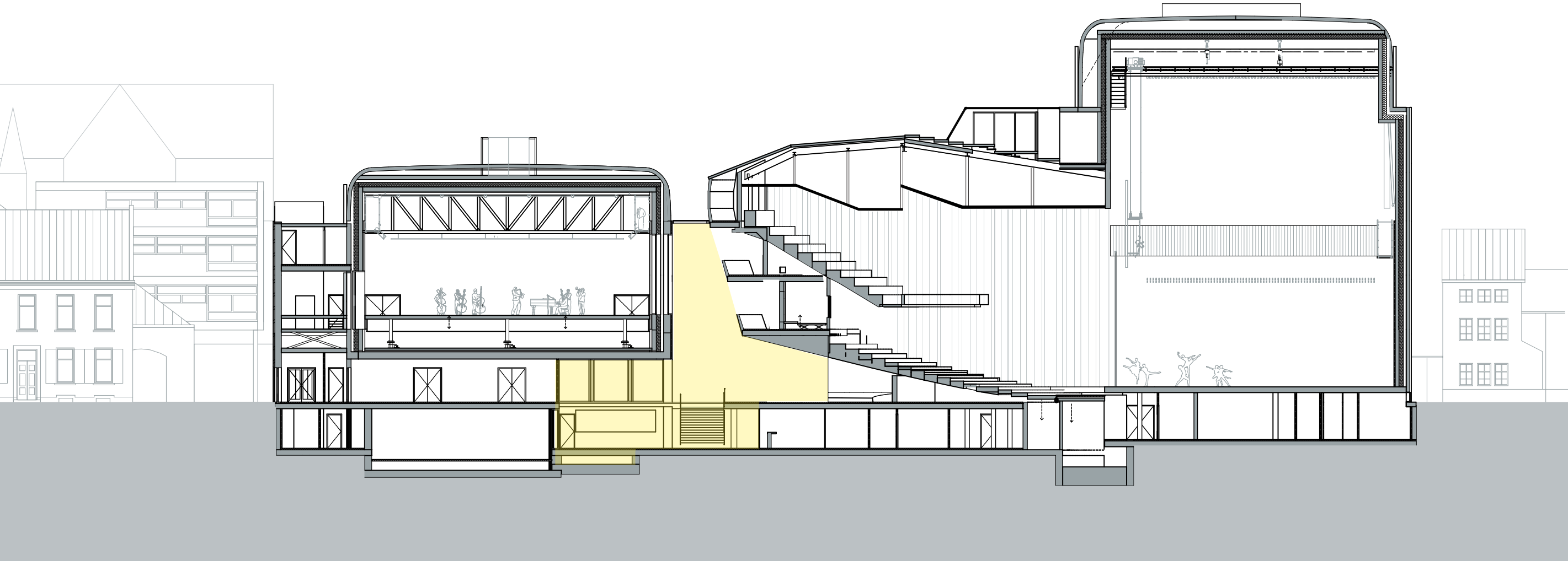
Doorsnede A-A
